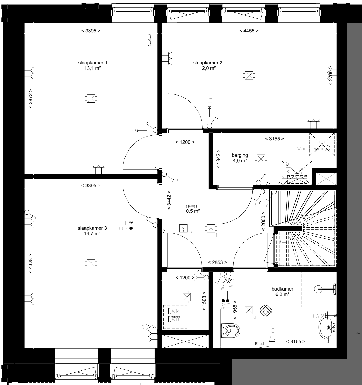
1e Verdieping
