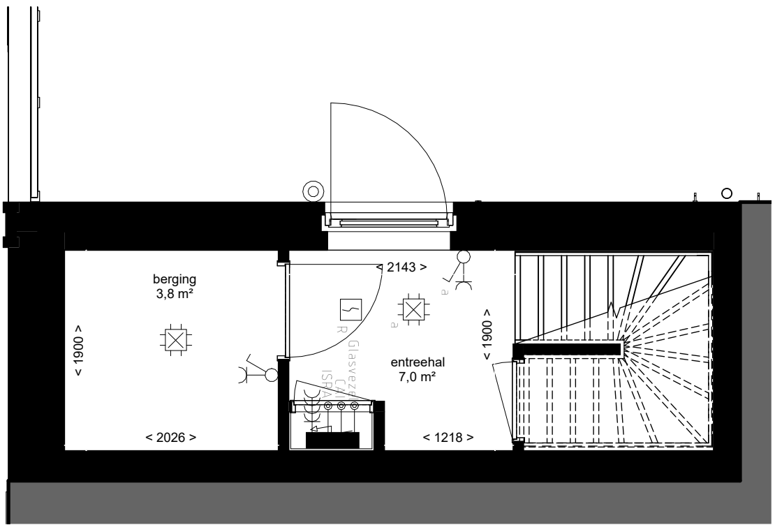
Begane grond
