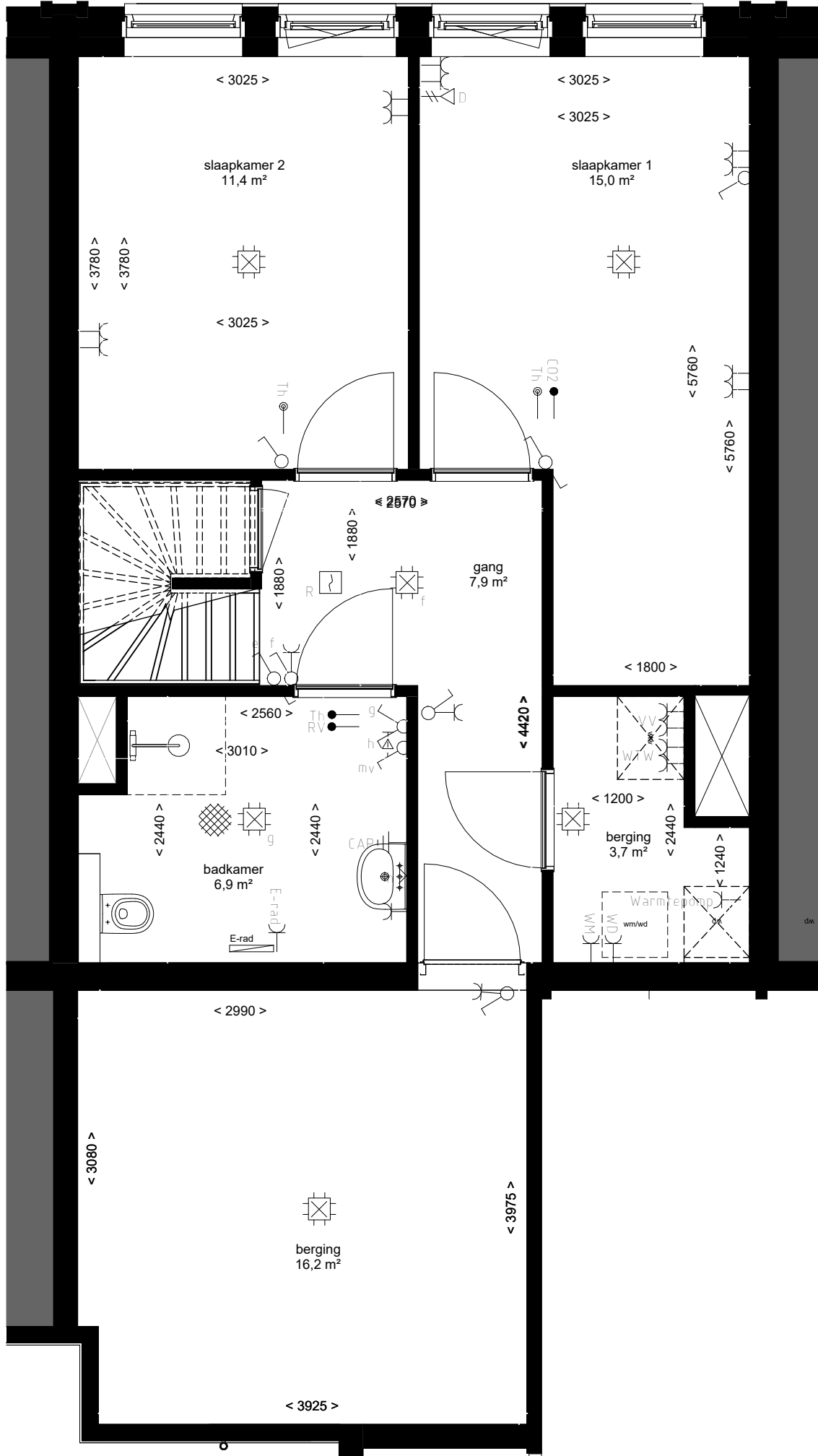
1e Verdieping
