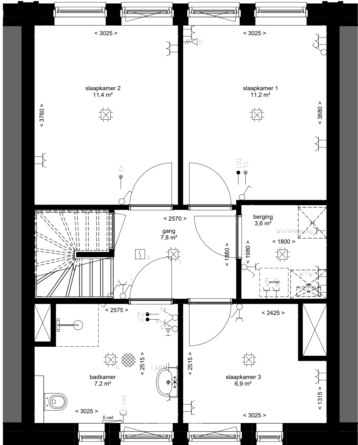
1e Verdieping
