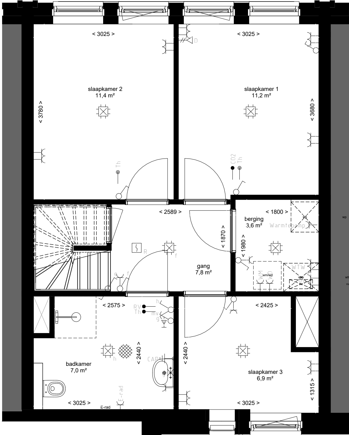
1e Verdieping
