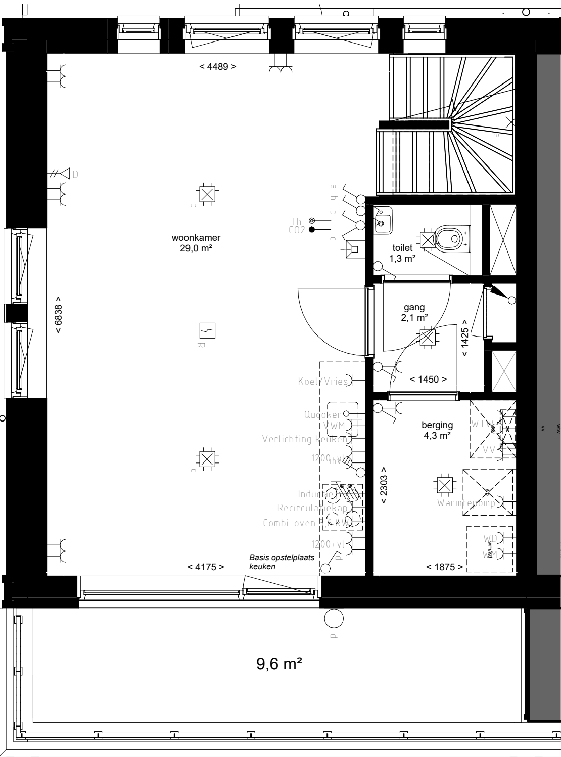
1e Verdieping
