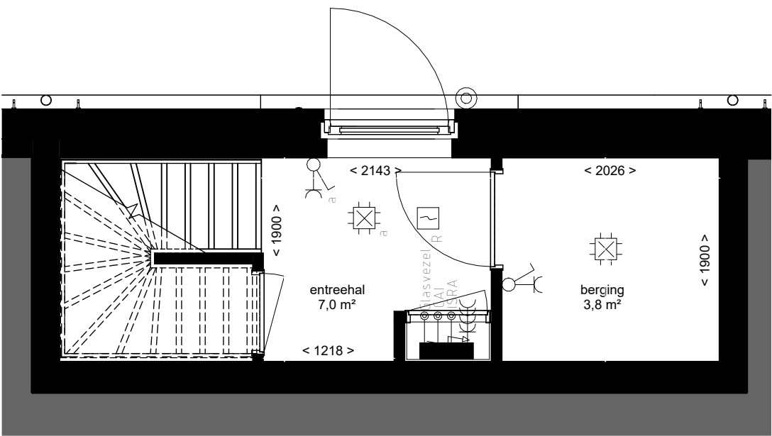
Begane grond
